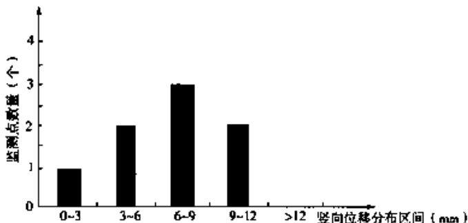
图1 桩顶竖向位移数据统计
